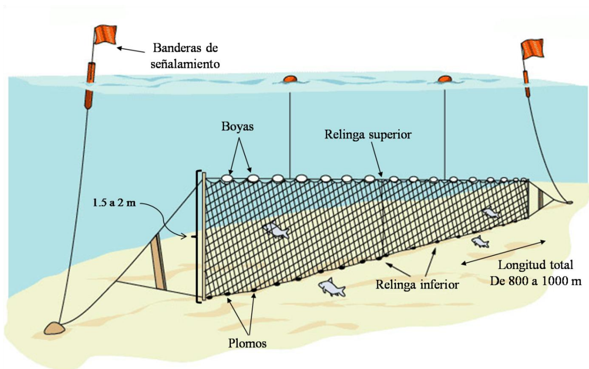
Figura 8. Características de las redes utilizadas por los pescadores artesanales de la costa occidental de B.C.S. Tomado de Michigan Sea Grant (2010) y modificado por el autor.
