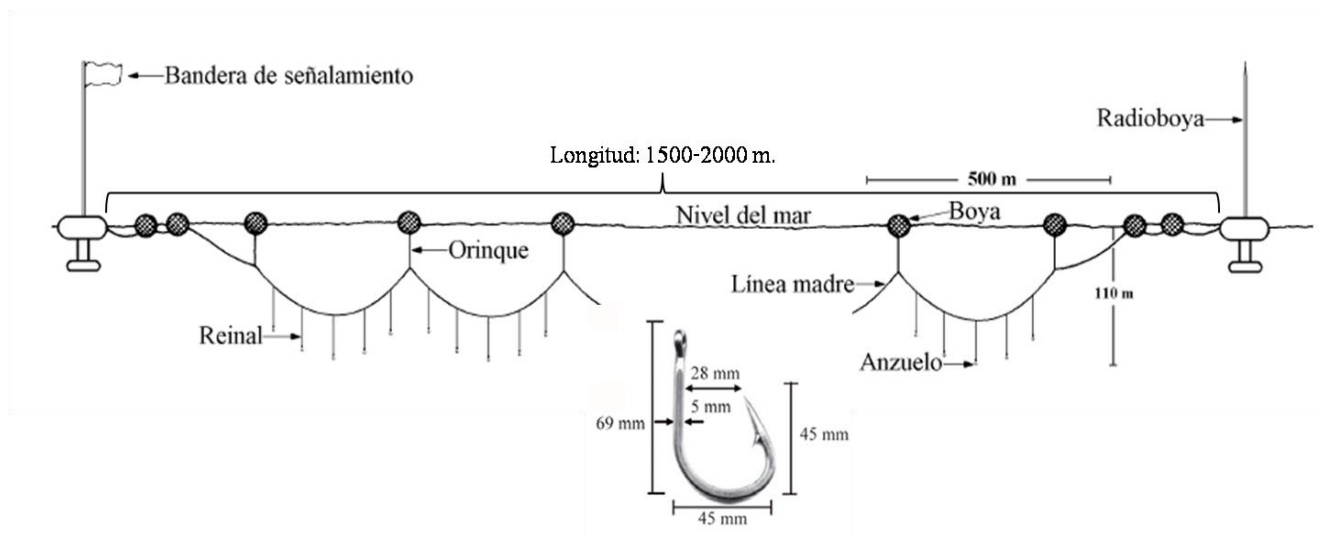
Figura 9. Características de las palangres y anzuelos utilizados por los pescadores artesanales de la costa occidental de B.C.S. Tomado de Santana-Hernández (2001) y modificado por el autor.
