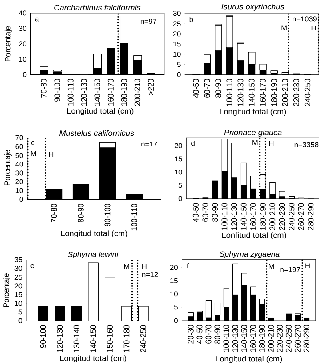
Figura 11. Distribución de frecuencia por sexo para los elasmobranquios capturados por palangres en la costa occidental de B.C.S. La n hace referencia al número de individuos medidos a partir de los cuales están basados los histogramas, y no necesariamente al número total de individuos capturados. Las hembras están representadas con columnas negras, los machos por las columnas blancas y los individuos indiferenciados por las columnas grises. Las líneas punteadas indican la talla de primera madurez de acuerdo a los siguientes autores: Ebert, (2003) (c,f), Hoyos-Padilla, (2003) (a); Shoou-Jeng y Hua-Hsun, (2005) (b); Carrera-Fernández et al. , (2010) (d); Bejarano-Álvarez et al. , (2010) (e). En los casos donde exista una diferencia sustancial en la talla de primera madurez entre sexos las líneas se denominaron M (Machos) o H (Hembras).
