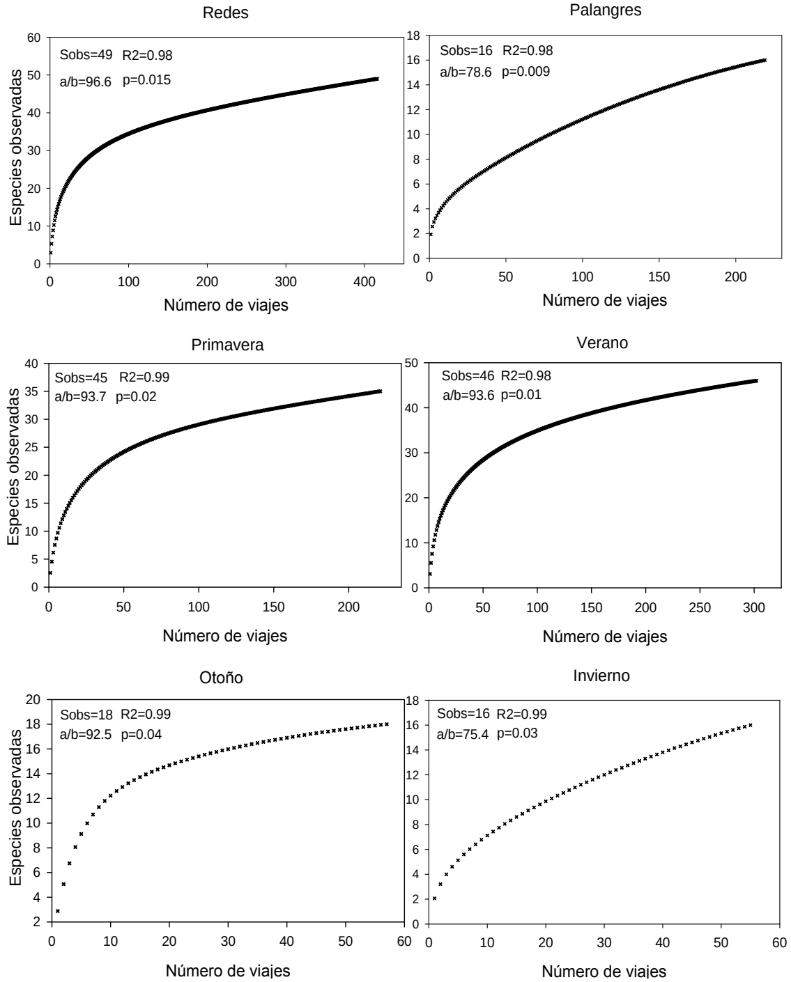
Figura 12. Curvas acumulativas para las especies de elasmobranquios, por artes de pesca (redes y palangres) y por temporadas de pesca (primavera, verano, otoño e invierno), de acuerdo al número de viajes muestreados. Donde Sobs=especies observadas, p=pendiente.
