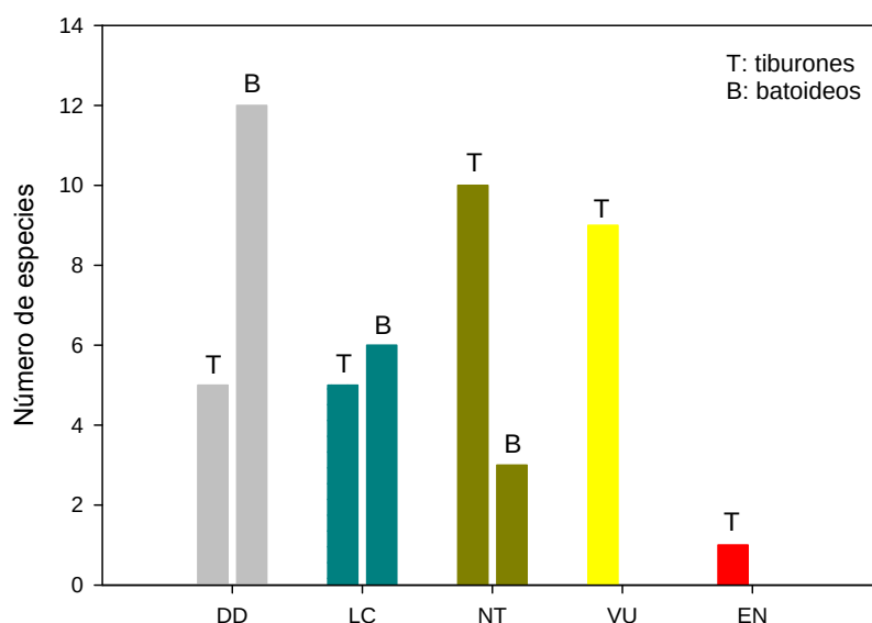
Figura 13. Categorías de la UICN para las especies de elasmobranquios registradas en la costa occidental de B.C.S. Abreviaturas: DD: Datos Insuficientes; LC: Preocupación Menor; NT: Casi Amenazado; VU: Vulnerable; EN: En Peligro.
