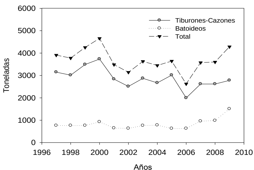
Figura 14. Capturas históricas de elasmobranquios en Baja California Sur de 1997 a 2009.
