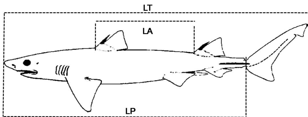
Figura 4. Medidas tomadas para los tiburones.
