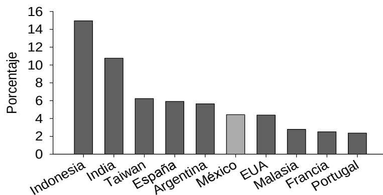
Figura 1. Países con mayor captura de elasmobranquios durante el 2007, (FAO, 2009).
