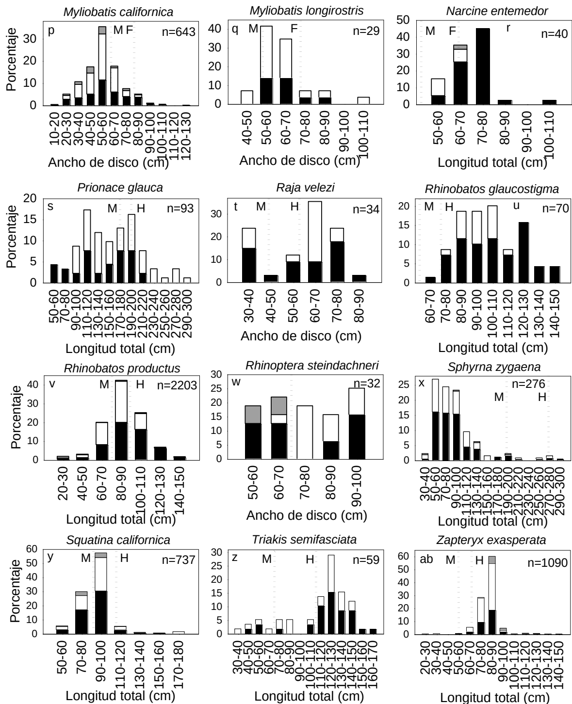
Figura 10. Distribución de frecuencia por sexo para los elasmobranquios capturados con redes en la costa occidental de B.C.S. La n hace referencia al número de individuos medidos a partir de los cuales están basados los histogramas, y no necesariamente al número total de individuos capturados. Las hembras están representadas con columnas negras, los machos por las columnas blancas y los individuos indiferenciados por las columnas grises. Las líneas punteadas indican la talla de primera madurez de acuerdo a los siguientes autores: Ebert, (2003) (a,c,d,e,g,h,i,L,n,p,v,x,z); Hoyos-Padilla, (2003) (b); Villavicencio-Garayzar et al. , (1994) (f); Compagno, (2001) (j); Shoou-Jeng y Hua-Hsun,
