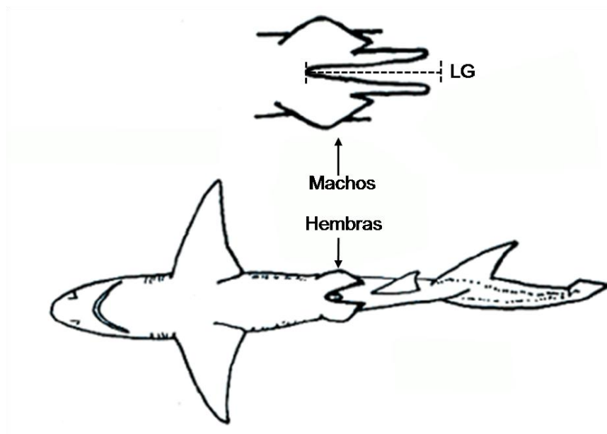
Figura 6. Diferenciación sexual y medida del gonopterigio en los machos.
