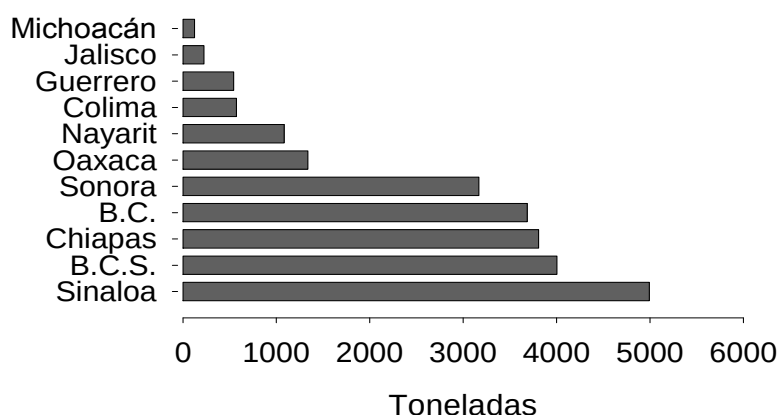
Figura 2. Captura de elasmobranquios en el Pacífico mexicano en 2009 (SAGARPA, 2009).
