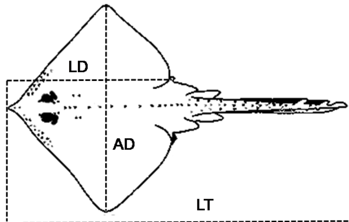
Figura 5. Medidas tomadas para los batoides.
