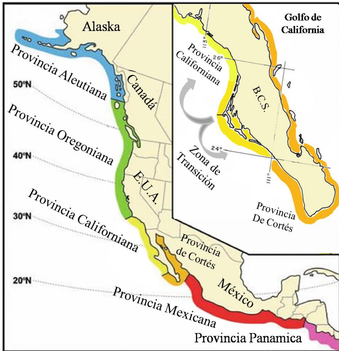
Figura 15. Mapa biogeográfico de la costa occidental de Norteamérica, tomado de Horn et al. , 2006 y modificado por el autor.
